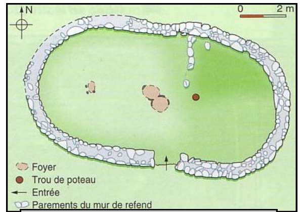
Document 2 : Plan des fouilles d'une maison paysanne XII e siècle en Bretagne - « Terre d'histoire » - Bordas
